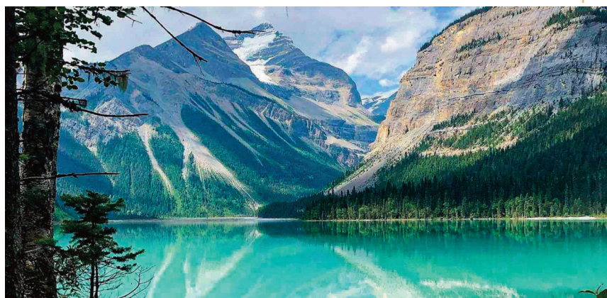
Les lacs des montagnes Rocheuses, de beaux exemples de lacs d'origine glaciaire
